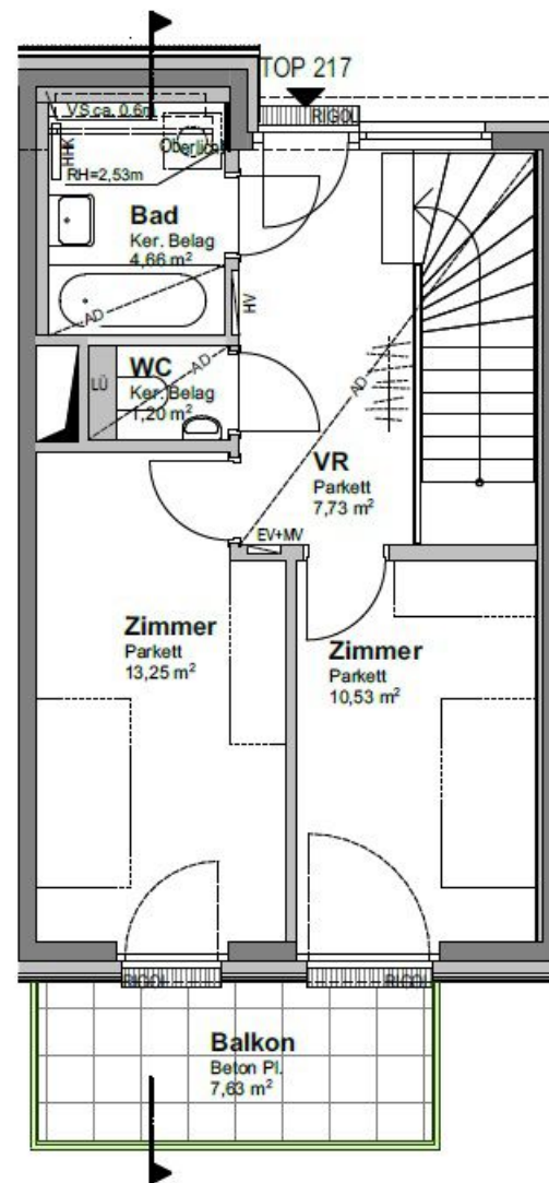
1. OBERGESCHOSS
