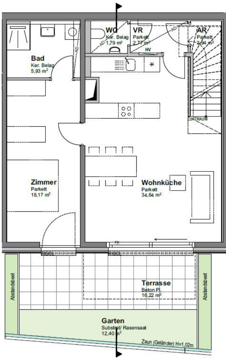
ERDGESCHOSS
